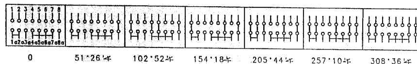
SCHEMA CONTATTI DEL COMMUTATORE FORNO mod. S600
